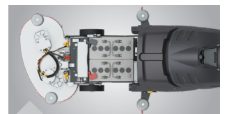
Bürstenköpfe austauschbar, dadurch nur eine Maschine mit unterschiedlichen Bürstenköpfen verwendbar statt verschiedene Maschinen
