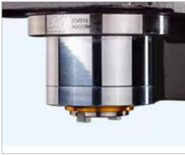
Frässpindeln mit 10.000 UpM
