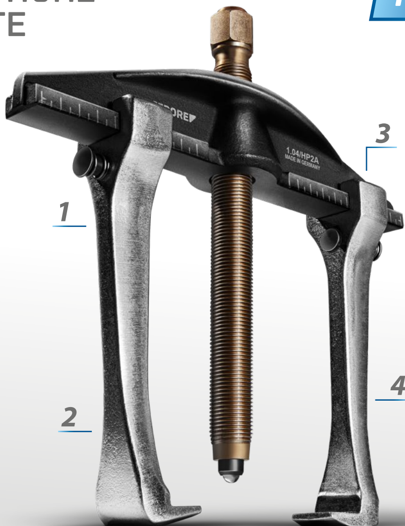
2-Arm High Power inkl. Hydraulik & Schutzfolie - 1.04/HP2A-B-HSP1-S
