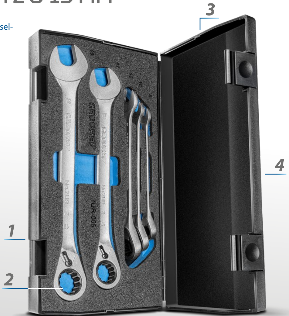
Satz Maulschlüssel mit Ringratsche 5-teilig - 7 UR-005
