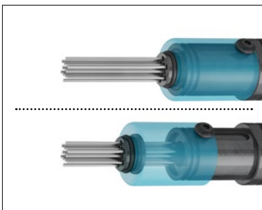
Verstellbarer Nadelschlitten mit integrierter Nadelführung gewährleistet lange Standzeiten
