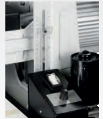
Höhenverstellung der Schleifeinheit an einer Skala ablesbar
